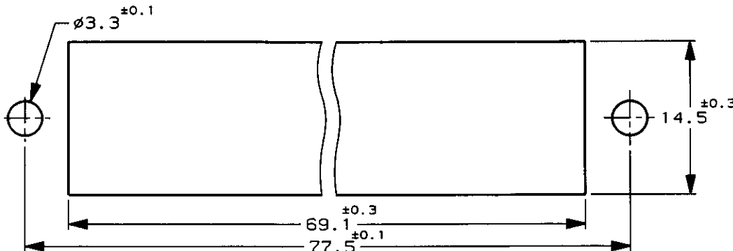
推奨パネルカット寸法 t=1.6 RECOMMENDED PANEL LAYOUT t=1.6
