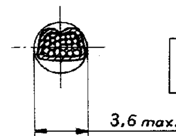
Schnitt C-D
