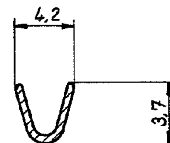
Schnitt A-B
