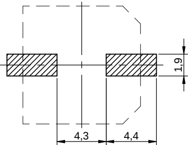
Scale - 2,5:1
