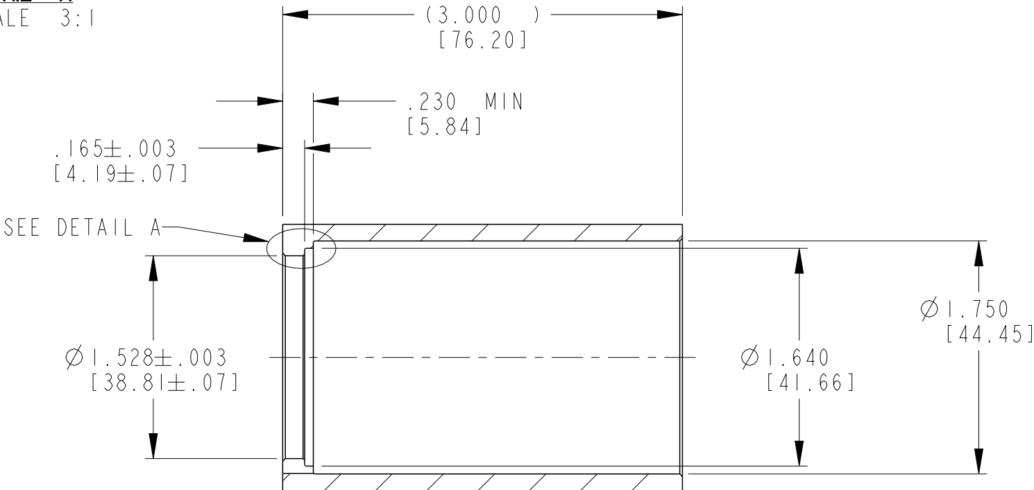
SECTION A-A
