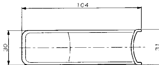
Abdeckkappe für 90°-Kabelabgang:
