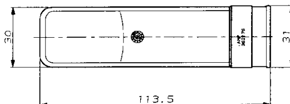
Abdeckkappe für 180°-Kabelabgang:
