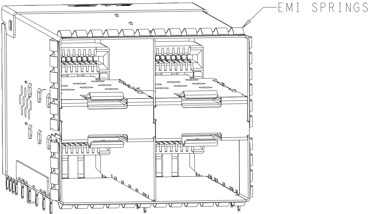
2343522-5 SCALE 3:1
