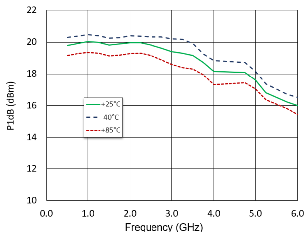
P1dB
