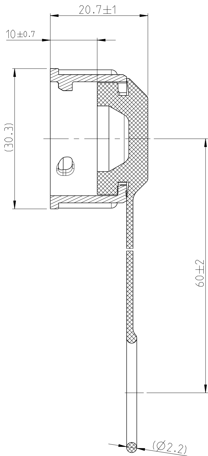
SECTION A-A
