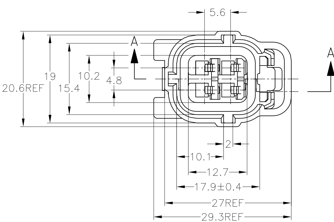
174257-2, 1-174257-2
