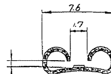
断面 A-A 尺度 8-1 (SECT) (SCALE)
